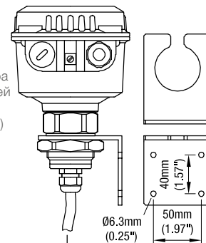
Поз.26 3-4 разнесенный корпус с монтажный уголок
