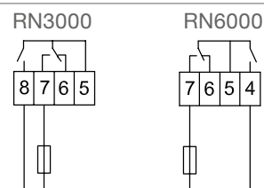
Сигнальный выход
