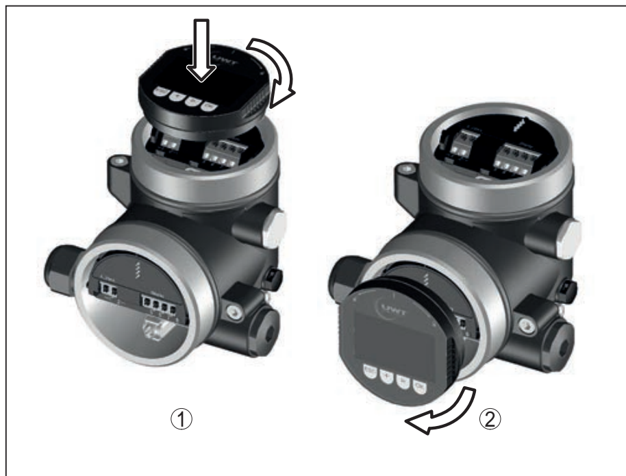
Рис. 11: Установка модуля индикации и настройки в двухкамерном корпусе
