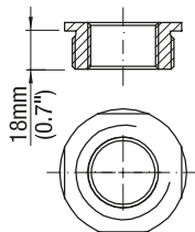
Адаптер G 1" к G 1 1/2"
